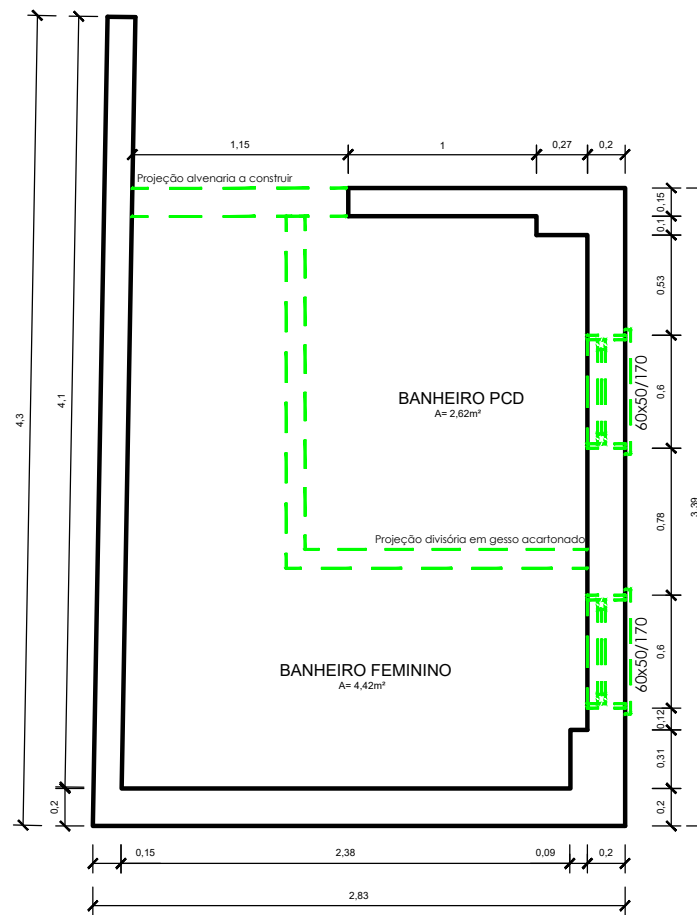
PLANTA BAIXA - A CONSTRUIR
