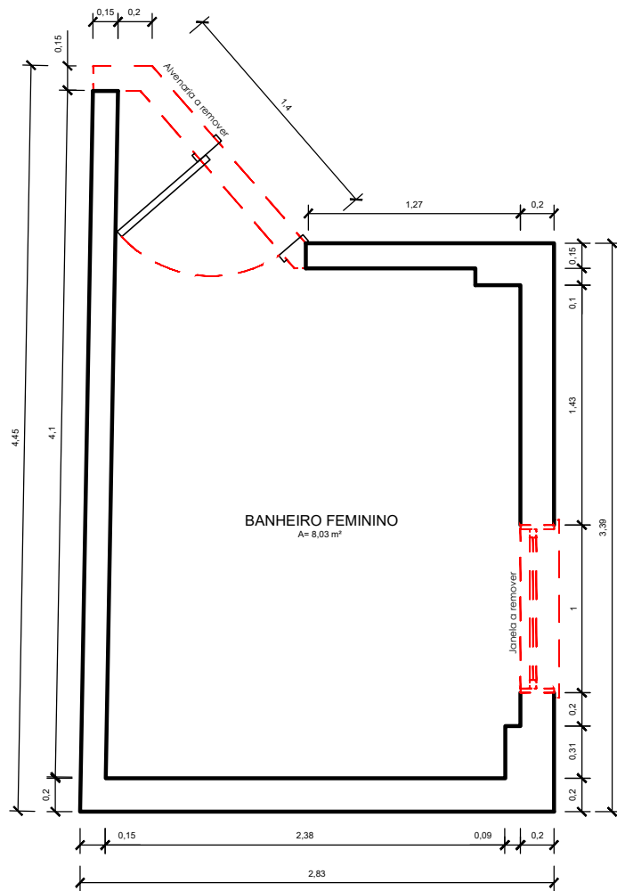
PLANTA BAIXA - A REMOVER
